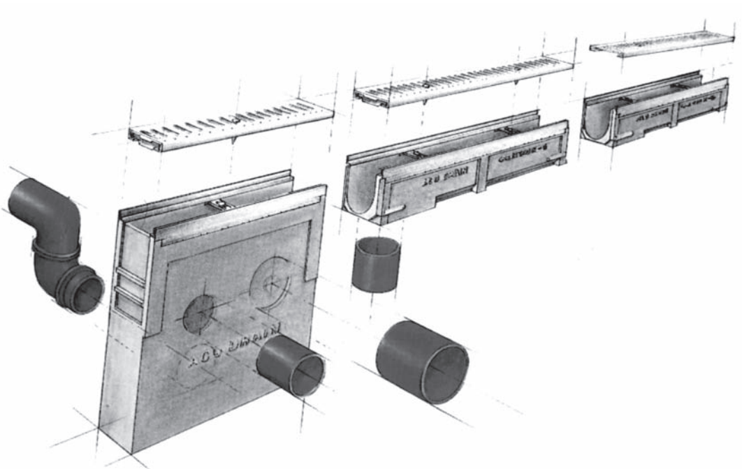
Overzicht ACO DRAIN® N 100 K met Quicklock®
